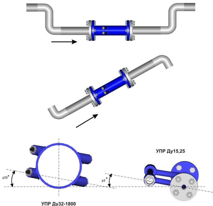
Рисунок 14 – Монтаж УПР на трубопроводе
