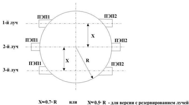
Рисунок 12 – Положение пар ПЭП для трехлучевых расходомеров
