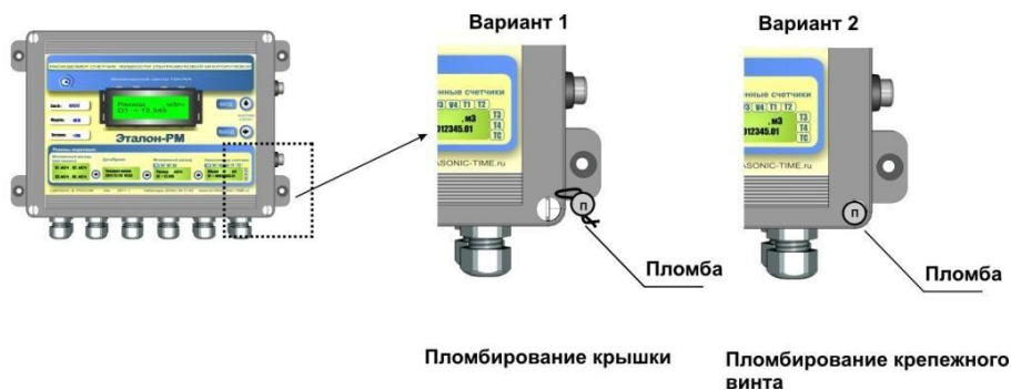
Рисунок 7 – Варианты пломбирования ЭБ
