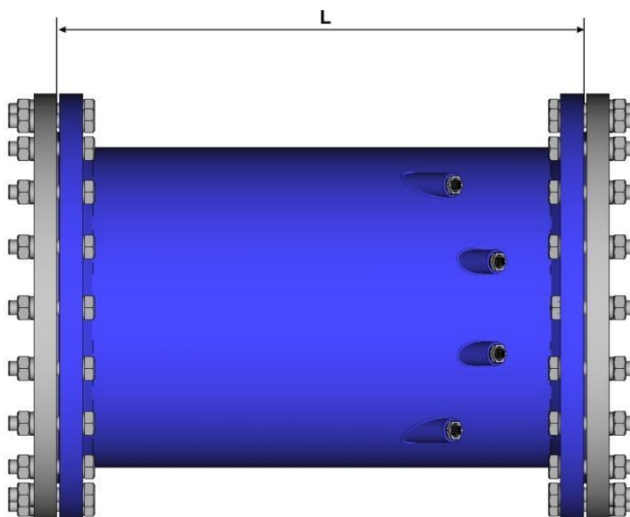
Рисунок 2 – Габаритные размеры и массы УПР
