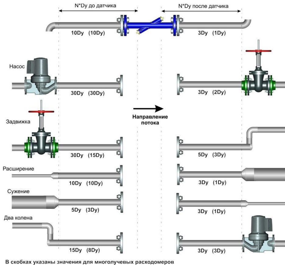
Рисунок 15 – Длины прямолинейных участков
