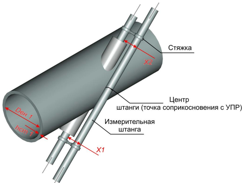
Рисунок 5 – Измерение смещения с помощью ПР005
