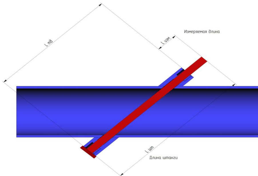
Рисунок 6 – Измерение длины L_a
