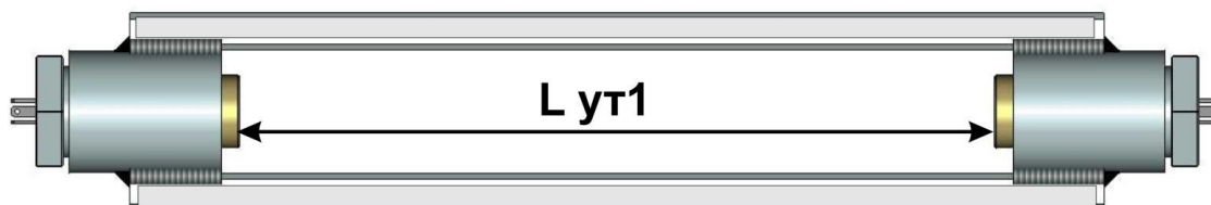
Рисунок 3 – Приспособление УТ-001
